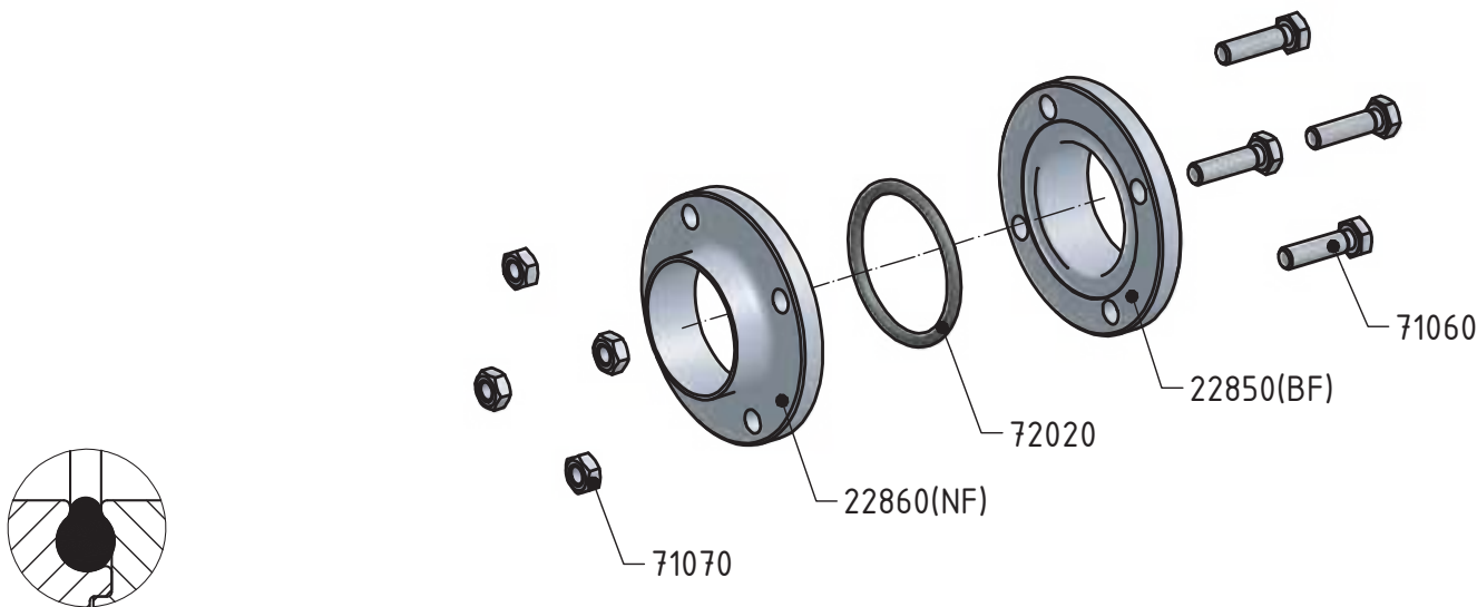
Деталь уплотнения
